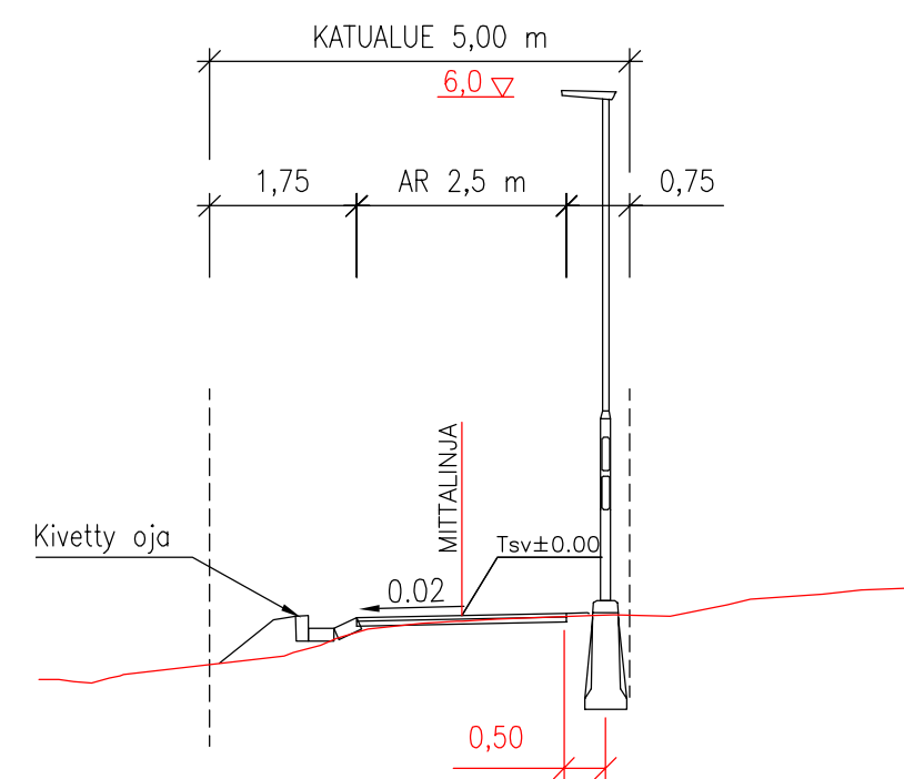
TYYPPIPOIKKILEIKKAUS 1:100 plv 102–116 (pl 115)
