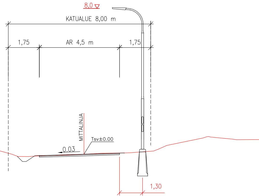
TYYPPIPOIKKILEIKKAUS 1:100 plv 8–80 (pl 50)
