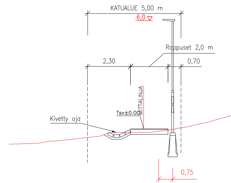
TYYPPIPOIKKILEIKKAUS 1:100 plv 90–102 (pl 95)
