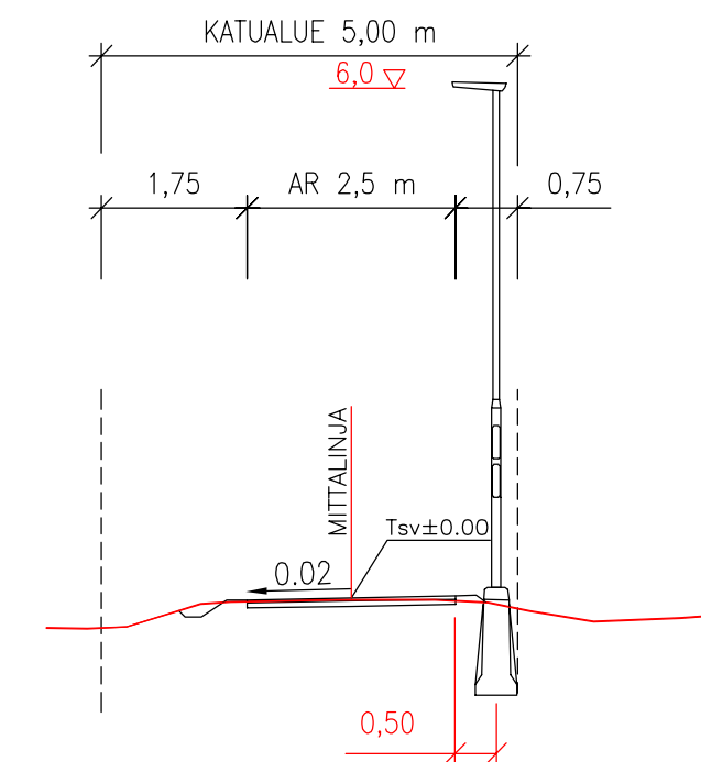
TYYPPIPOIKKILEIKKAUS 1:100 plv 116–144 (pl 130)
